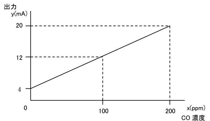
図 12 CO 濃度対アナログ出力の関係
