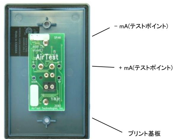
図 10 プリント基板とテストポイント
