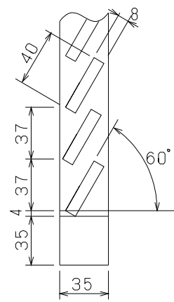
B部詳細図(1/2)
